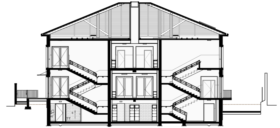
Corte C
