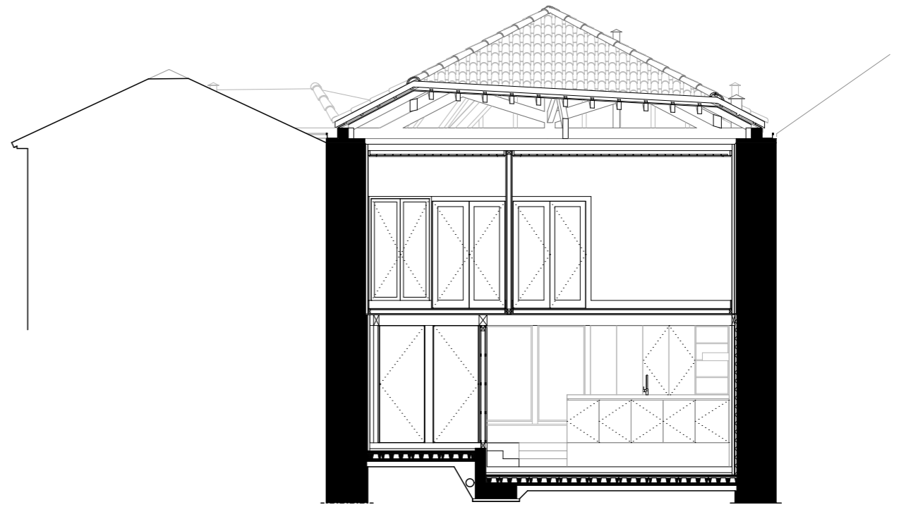
Corte transversal
