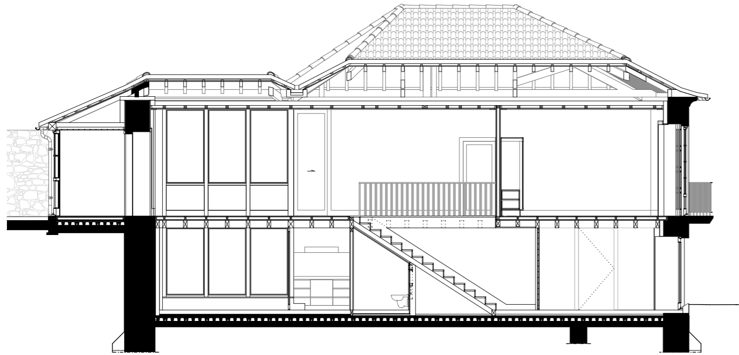
Corte longitudinal
