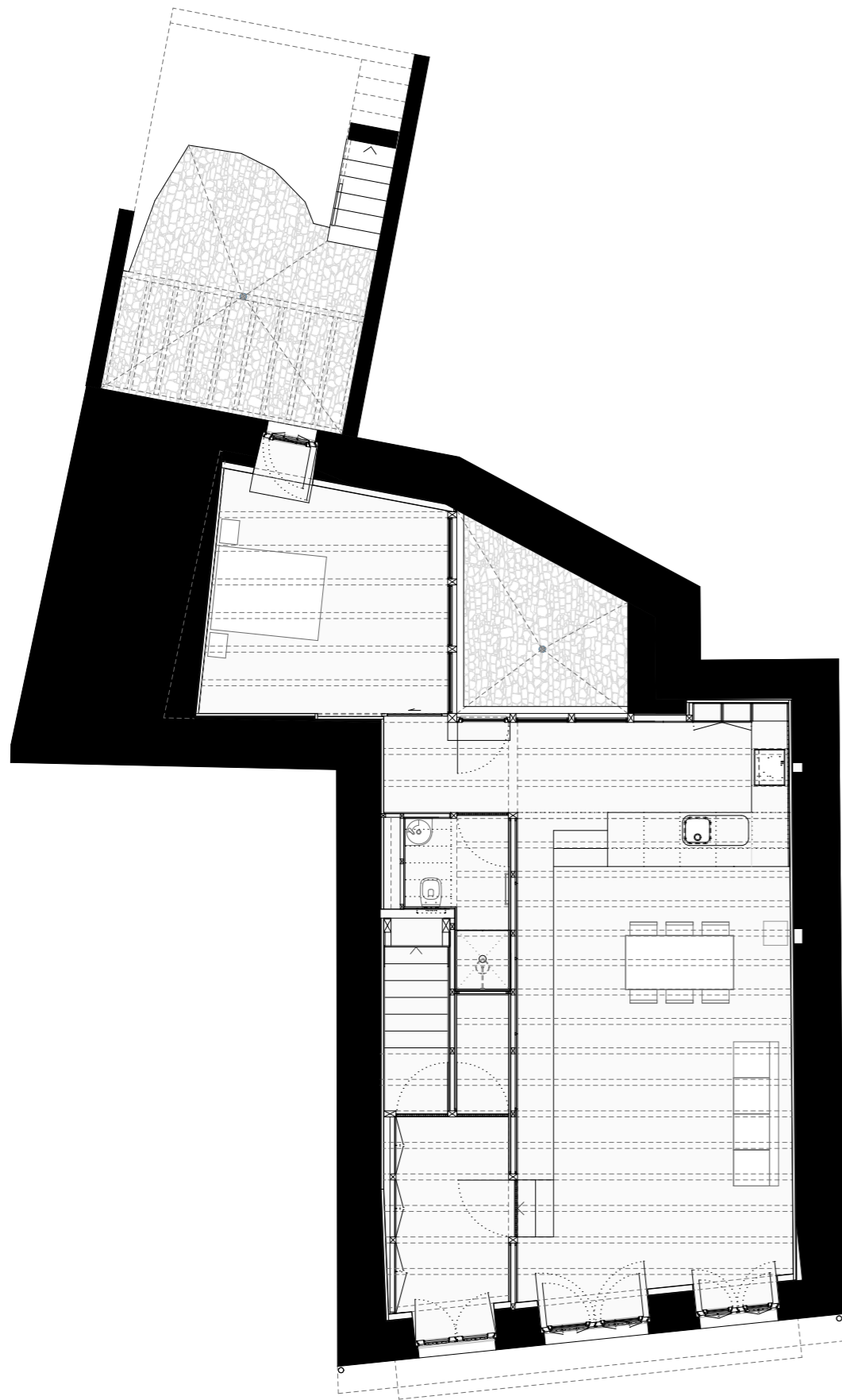
Planta Piso 0
